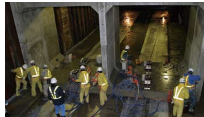
連結施工例 (2 函体連結) [w=67.4t]
